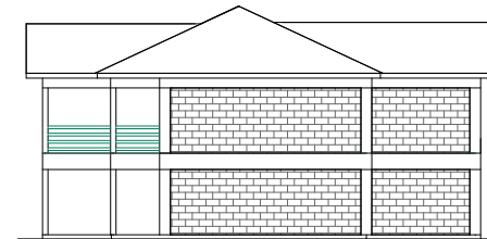
ELEVATION 04
