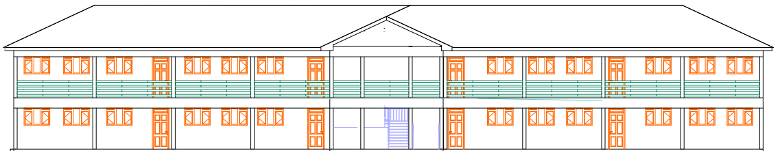
ELEVATION 01
