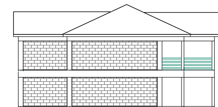
ELEVATION 02
